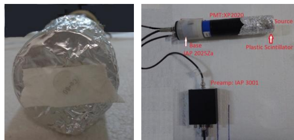
شکل (۳): نمونه سوسوزن مونتاژ شده روی PMT و نحوه قرارگیری چشمه روی سوسوزن.
