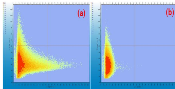
شکل (۱۰): طیف سه پارامتری (انرژی، زمان، شمارش) از چشمه نوترون ^{252}\text{Cf} و چشمه گاما ^{137}\text{Cs} .
