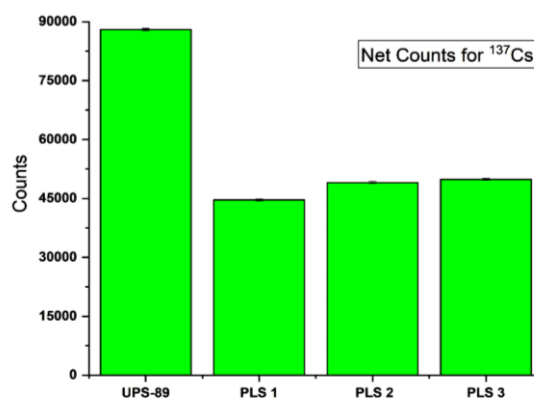
شکل (۷): مقایسه مقدار انتگرال سطح زیر طیف هر نمونه برای چشمه 137 Cs.
