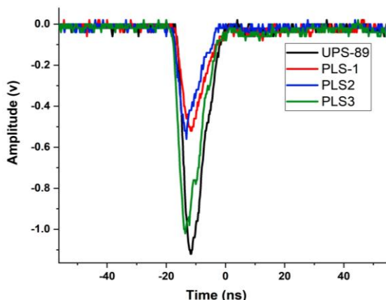
شکل (۹): نمونه پالس آند سوسوزن‌ها.
