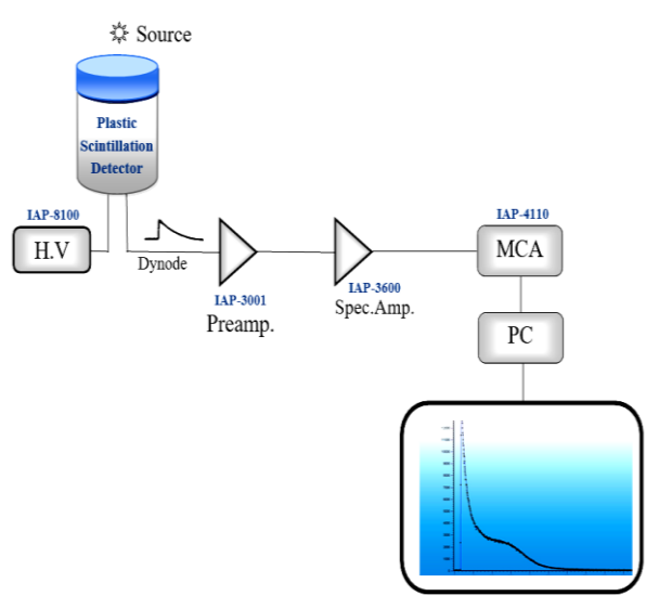
شکل (۲): چیدمان طیف‌نگاری با استفاده از سوسوزن‌های پلاستیک.
