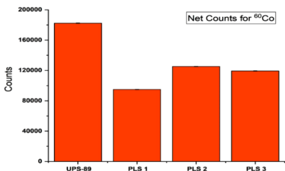
شکل (۸): مقایسه مقدار انتگرال سطح زیر طیف هر نمونه برای چشمه 60 Co.
