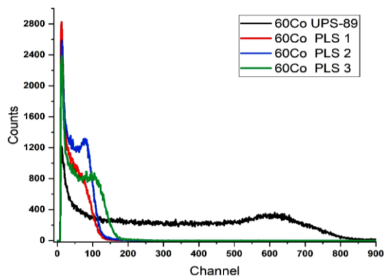
شکل (۶): پاسخ نسبی نمونه‌ها به چشمه 60 Co.
