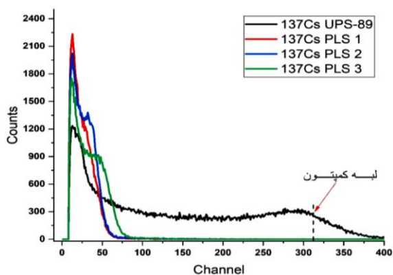
شکل (۵): پاسخ نسبی نمونه‌ها به چشمه ^{137}\text{Cs} .
