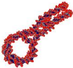
شکل (۱): مدل ۱ZBB (کره های قرمز پایه و کره های آبی طوسی رشته های اول و دوم DNA). توزیع یکنواخت الکترون ها در حجم پر از آب اطراف DNA.
