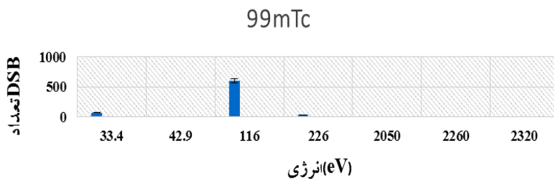
شکل (۴): تعداد DSBها در انرژی‌های طیف ^{99\text{m}}\text{Tc} .
