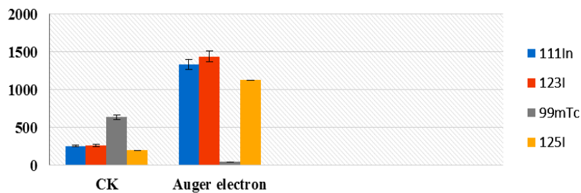
شکل (۷): مقایسه مقدار DSB الکترون اوژه و الکترون اوژه کاسترکرونینگ در ^{111}\text{In} ، ^{125}\text{I} ، ^{123}\text{I} و ^{99\text{m}}\text{Tc} .
