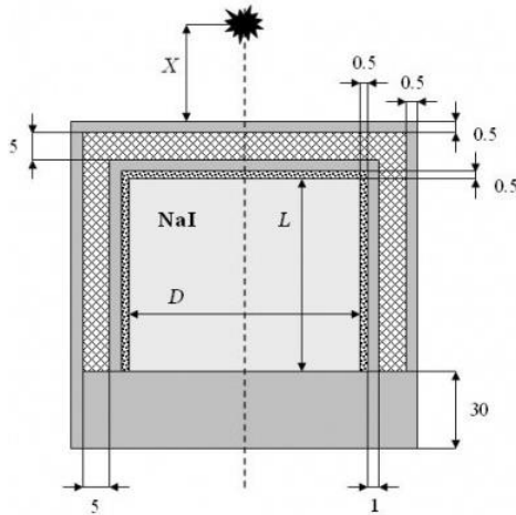
شکل (۱): طرح واره ساختار درونی آشکارساز 3'' \times 3'' NaI(Tl).
