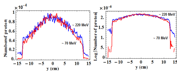
شکل (۵): مقایسه‌ی پروفایل تعداد پروتون‌ها به ازاء x=0 در یک فاصله (z) از چشمه و برای دو طیف انرژی مختلف.
