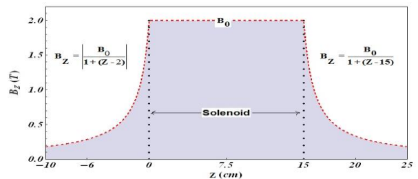
شکل (۲): نمایشی از الف) اجزاء سیم‌لوله و محل قرارگیری چشمه پروتونی و روزنه گزینش‌گر ذرات بعد از اعمال میدان مغناطیسی، ب) هندسه‌ی کامل سیم‌لوله‌ی شبیه‌سازی شده در دو جهت (ج) میدان مغناطیسی اعمال شده درون سیم‌لوله موردنظر.
