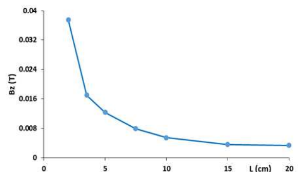
شکل (۶): میدان مغناطیسی محوری (راستای Z) با واحد تسلا بر حسب فاصله‌ی مغزه‌ها در نقطه‌ی (y = z = 0) .
