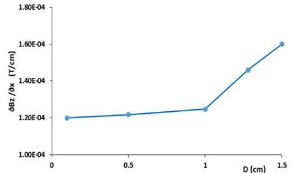
شکل (۵): گرادیان مولفه‌ی محوری (Z) میدان مغناطیسی در جهت X بر حسب قطر نوک مغزه‌ها در نقطه‌ی (y = z = 0) .
