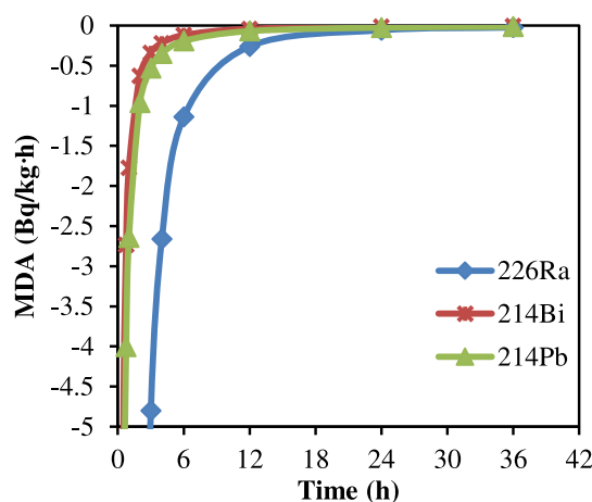
شکل (۷): مشق زمانی کمترین اکتیویته آشکار شده رادیونوکلیدهای سری ^{238}\text{U} .
