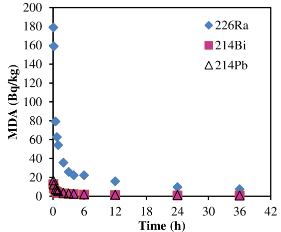
شکل (۳): تغییرات کمترین اکتیویته آشکار شده بر حسب زمان شمارش برای رادیونوکلیدهای ^{238}\text{U} .
