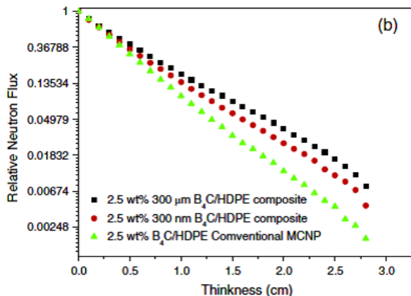
شکل (۱): مقایسه جذب نوترون حرارتی برای 300\mu m و 300\text{ nm} ذرات کاربرد بور و محاسبات معمول MCNP.
