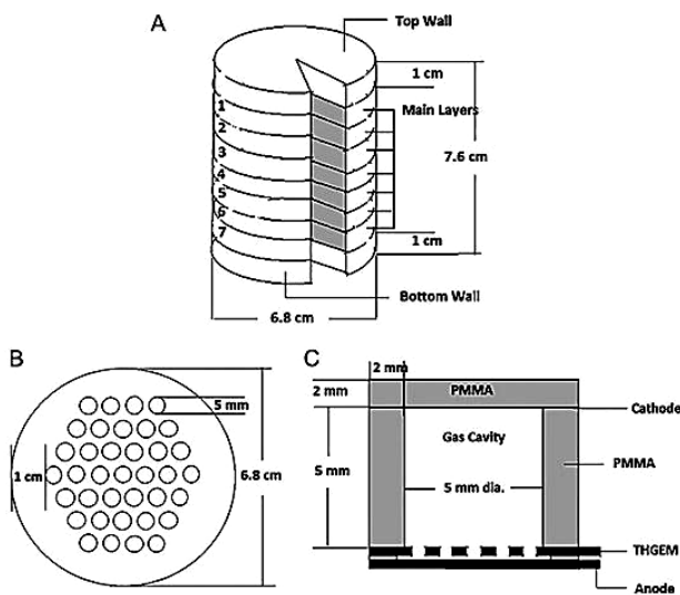
شکل (۱): آشکارساز میکرودمتری طراحی شده [۱۲].
