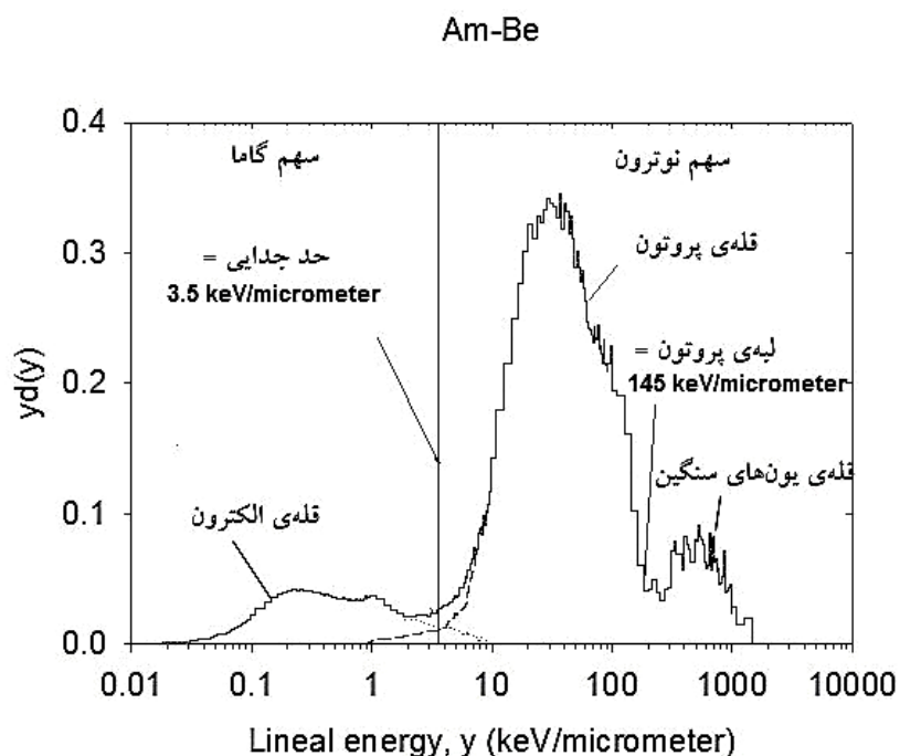
شکل (۳): منحنی بهنجار توزیع انرژی خطی میدان آمیخته‌ی نوترون-گامای چشمه‌ی ^{241}\text{Am} -Be.
