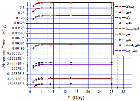
شکل (۵): نمودار دز جذب شده در بافت‌های مختلف بدن حاصل از پرتوهای گاما گسیل شده از استنت پرتوزای ^{188}\text{Re} با فعالیت اولیه 1\ \mu\text{Ci} پس از گذشت ۲۸ روز.
