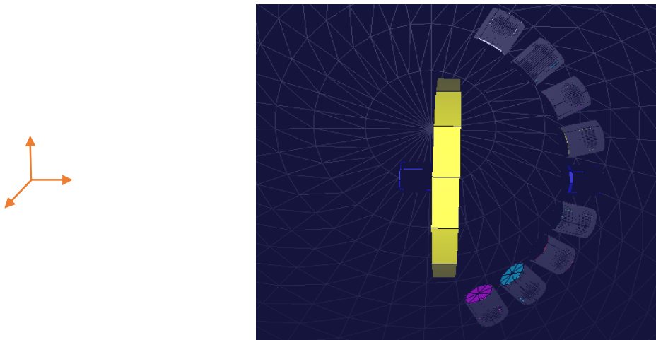
شکل (۲): توزیع زاویه‌ای آشکارساز CSI(TI) در حضور چشمه فوتونی ( ^{137}\text{Cs} ، ^{60}\text{Co} و ^{16}\text{N} ) و لایه حفاظی فوتون (سرب، آهن و آلومینیوم) جهت بررسی اثر مکان آشکارساز روی ضریب انباشت.
