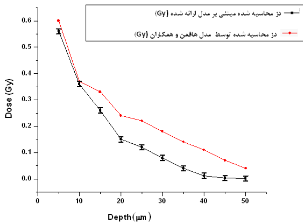
شکل (۵): مقایسه تغییرات دز محاسبه شده مبتنی بر شار برای WLM
