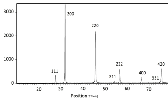
شکل (۱): نمودار XRD ذرات NaCl.
