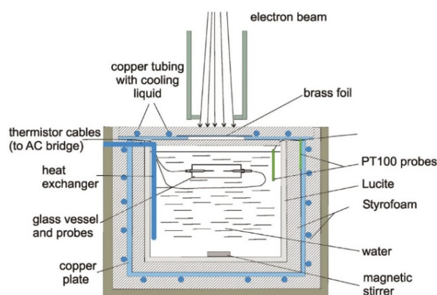
شکل ۱: طراحی کلی از یک کالریمتر آب نوعی [۵]
