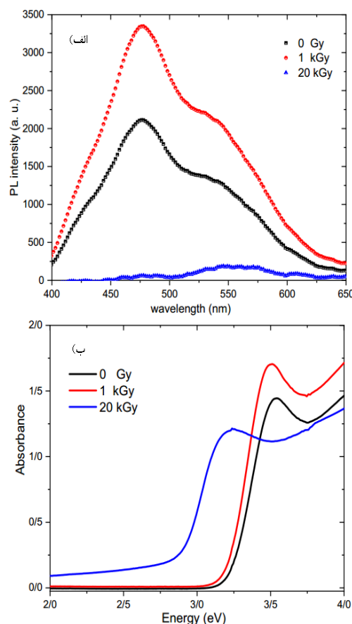
شکل (۲): (الف) طیف فوتولومینسانس و (ب) طیف جذبی نقاط
