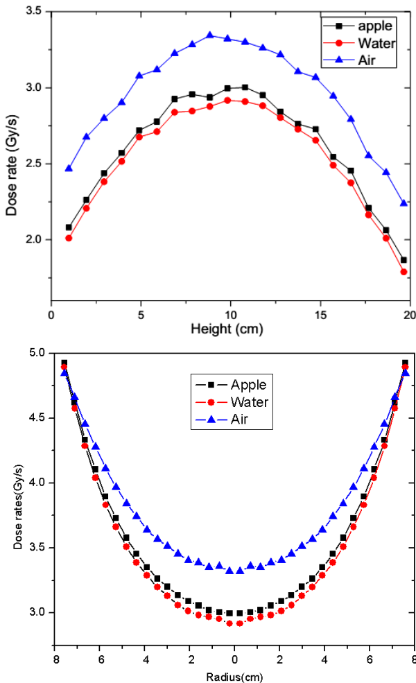
شکل (۳): منحنی‌های برشی محوری (بالا) و شعاعی (پایین) آهنگ دز در سه محیط هوا، سیب و آب.
