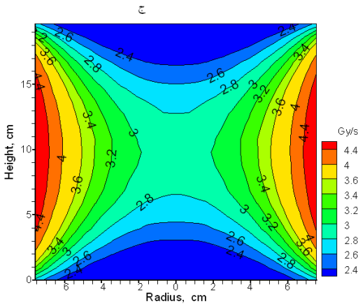
شکل (۲): منحنی‌های هم دز در هوا (الف)، سیب (ب) و آب (ج). محور افقی راستای شعاعی و محور عمودی راستای محوری گاما سل را نشان می‌دهد. اعداد بر روی منحنی‌ها مقادیر آهنگ دز بر حسب Gy/s است.
