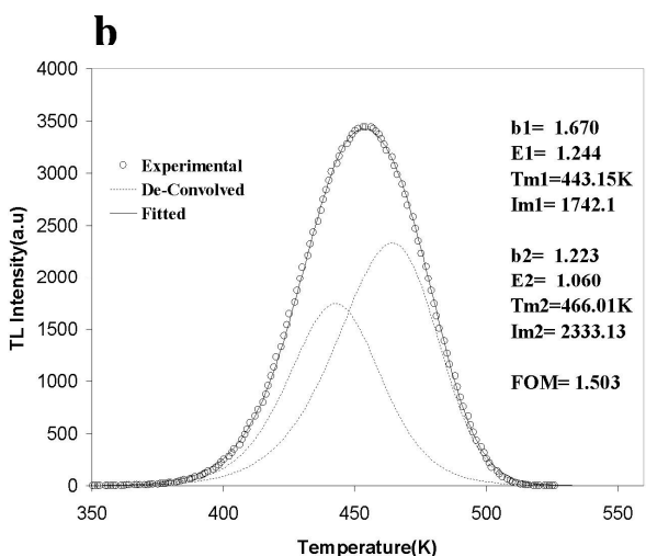
شکل ۲: منحنی برازش شده دزیمتر \alpha\text{-Al}_2\text{O}_3\text{:C} در پرتودهی (a) ۴۰ msv و ۹ گاما و ۴۰ msv نوترون (b) در پرتودهی ۱۷ msv گاما و ۴۰ msv نوترون. پارامترهای گیراندازی به دست آمده از برازش انجام شده در شکل مشاهده می‌شود.
