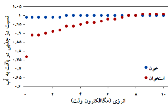
شکل (۵): تغییرات نسبت دز جذبی در بافت به آب بر حسب انرژی فرودی که با استفاده از روش تحلیلی محاسبه شده است.
