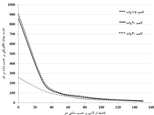
شکل (۹): نمودار تغییرات شدت میدان الکتریکی در فرکانس ۵۰ هرتز با تغییر فاصله از CFLها.
