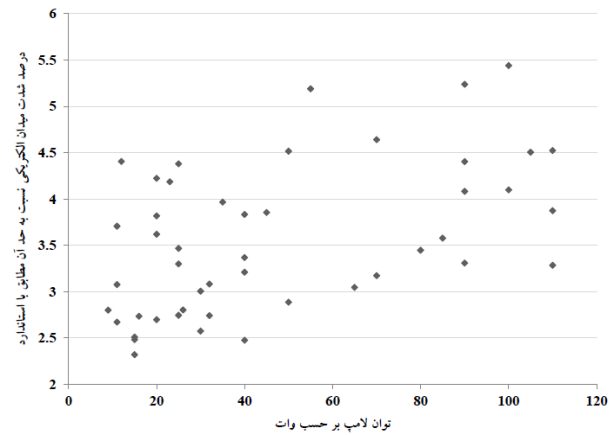
شکل (۸): نمودار تغییرات درصد شدت میدان الکتریکی در فرکانس ۵۰ هرتز و فاصله ۳۰ سانتی متری CFLها به حد شدت میدان الکتریکی.
