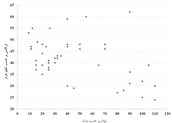
شکل (۶): فرکانس بالاست برای CFLها با توان‌های مختلف.
