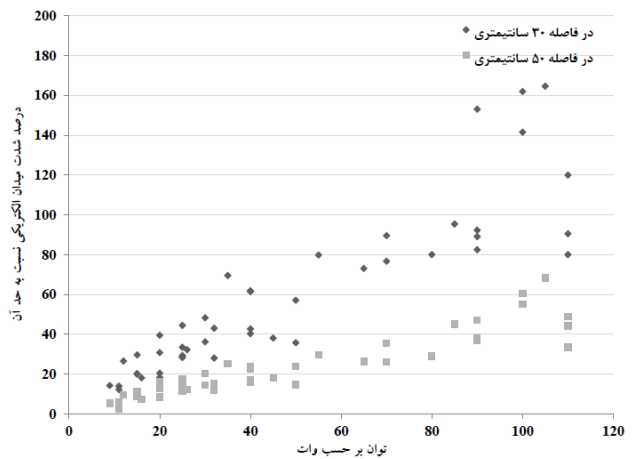
شکل (۱۱): نمودار تغییرات درصد شدت میدان الکتریکی در فرکانس کار بالاست و فاصله ۳۰ سانتی متری CFLها به حد آن برای مردم طبق استاندارد ملی و رهنمود ICNIRP.
