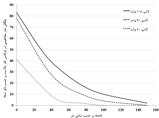
شکل (۱۵): نمودار تغییرات چگالی شار مغناطیسی در فرکانس کار بالاتر و فاصله ۳۰ سانتی متری از CFLها.
