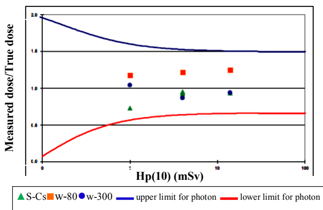
شکل (۳): نتایج دزیمتر فردی TLD فاز یک در مقایسه با نمودار شیپوری.
