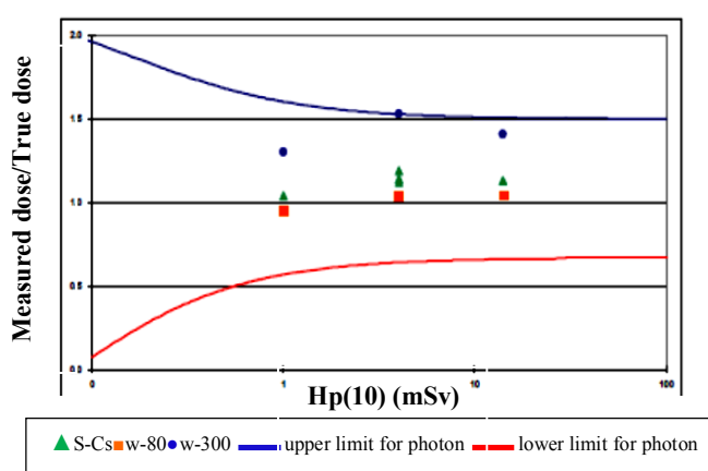
شکل (۲): نتایج دزیمتر فردی فیلم بچ فاز یک در مقایسه با نمودار شیپوری.
