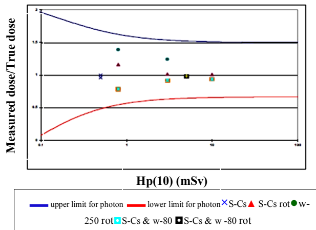
شکل (۴): نتایج دزیمتر فردی فیلم بچ فاز دو در مقایسه با نمودار شیپوری.
