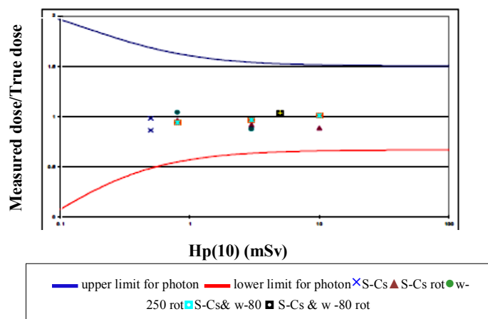
شکل (۵): نتایج دزیمتر فردی TLD فاز دو در مقایسه با نمودار شیپوری.
