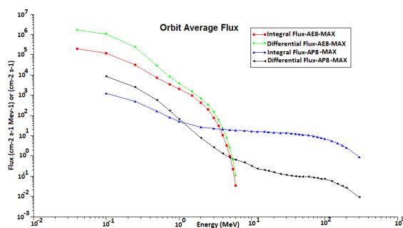
شکل (۲): میزان شار ذرات باردار موجود در کمر بند داخلی ون‌آلن
