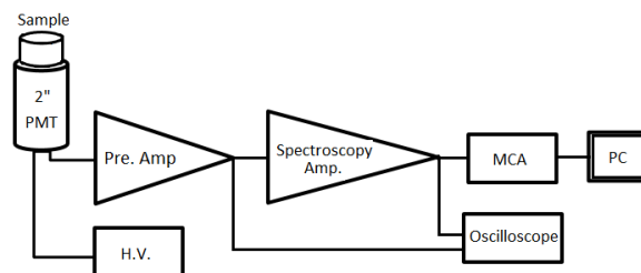
شکل (۱): چیدمان آزمایش اندازه‌گیری طیف ارتفاع پالس.
